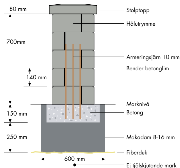
Sektionsritning stolpe 350 mm av Labyrint Mini. Används Labyrint Maxi blir stolpen 560 mm bred.
