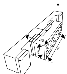
Bredd färdig mur 200 mm
