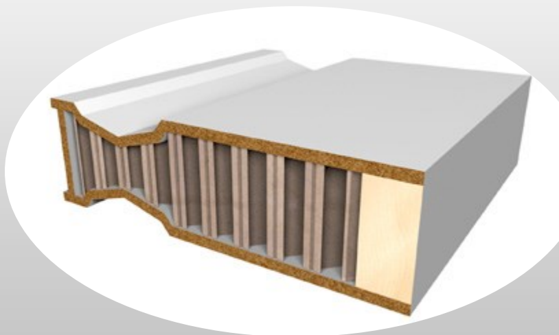
Detalj formpressad
