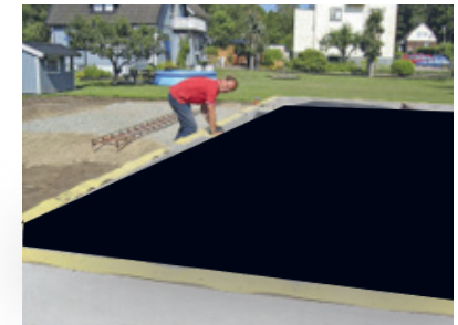
Radonmembran
